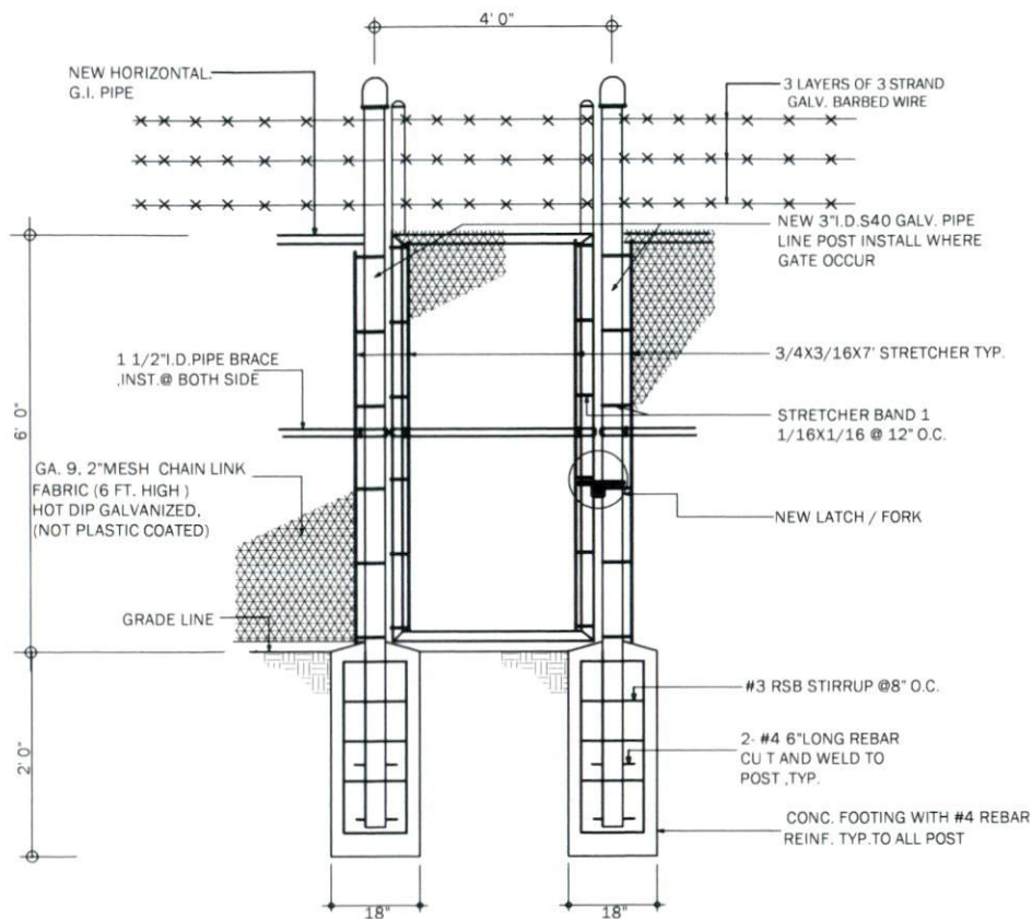
ACCESS GATE DETAIL N.T.S.
